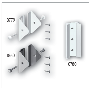
Edelstahl-Elementhalter
