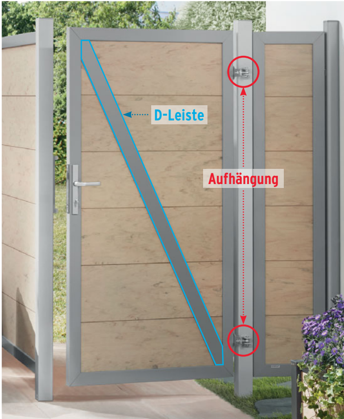
Art. 2443 DESIGN WPC ALU Tor DIN rechts im Farbton Sand. Die Profile der Tore sind in einem umlaufenden Metallrahmen verbaut. Die rückseitige Diagonalverstrebung aus Aluminium im Rahmenfarbton Silber (D-Leiste) bringt zusätzliche Stabilität. Metalltorpfosten mit angeschweißter Aufhängung (Seite 39).
