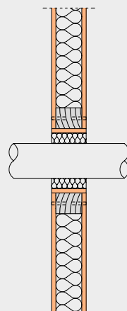
Rauchrohrdurchführung
