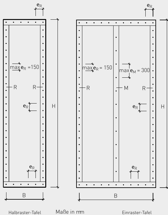
Bild 4+5: Maximal-Abstände der Befestigungsmittel mit fermacell® Gipsfaser-Platten
