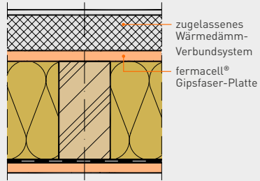
Wirksamer Wetterschutz WDVS
