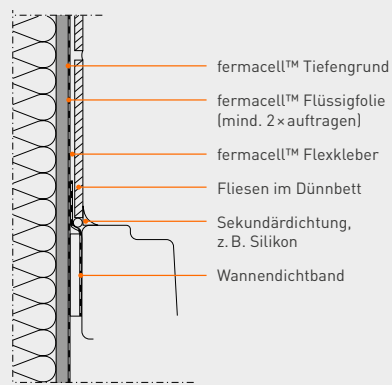
Anschluss Duschtasse-Wand mit Schalldämmstreifen
