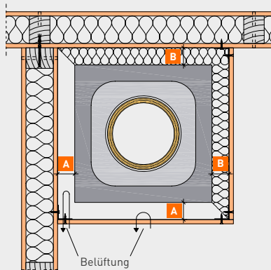
Schornstein mit Bekleidung vor Holztafelbauwand
