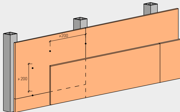
Versetzen der zweiten Lage bei mehrlagiger Beplankung
