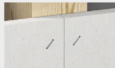
Platten stumpf gestoßen
