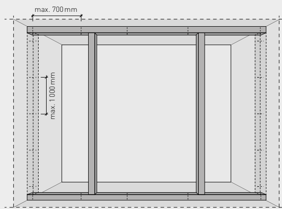
Befestigungsabstände
