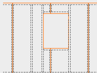
Fensteröffnung bei Fugenversatz
