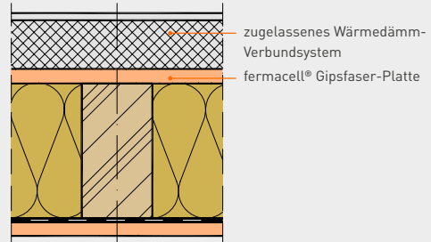
Dauerhaft wirksamer Wetterschutz WDVS
