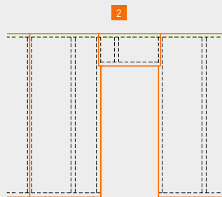
Türöffnung bei vertikalem Beplankungsstoß ohne Fugenversatz
