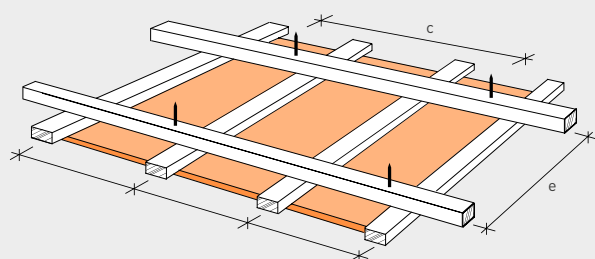
Grundlatte, direkt befestigt
