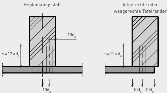
Bild 4: Erforderliche Randabstände für Klammern
