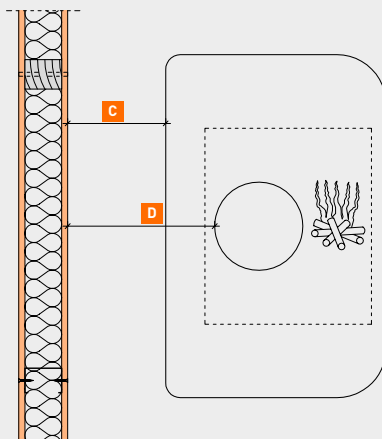
Abstände Öfen vor Holztafelbauwand
