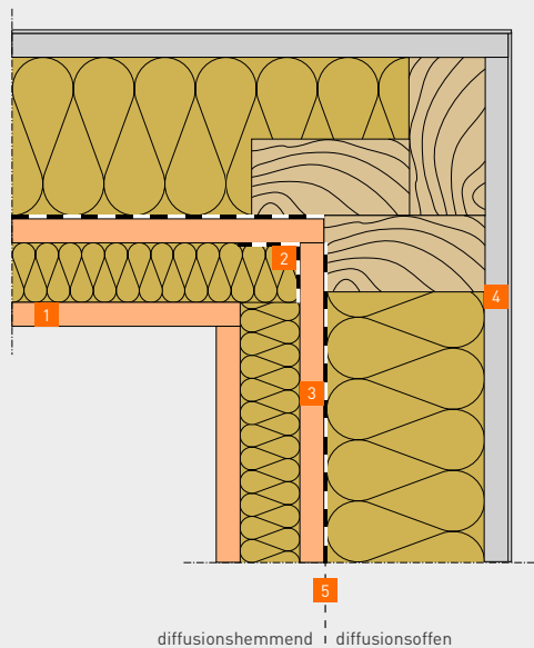
Luftdichte Ausführung - Außenecke Holztafelwände mit Installationsebene
