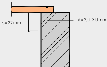
Bild 2: Sondernägel
