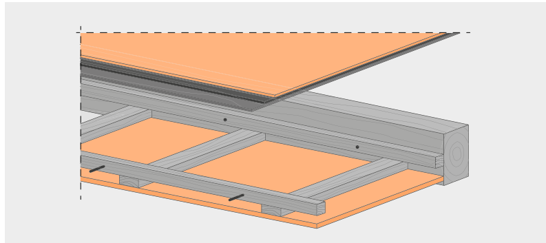
Befestigung mit Holz-Unterkonstruktion
