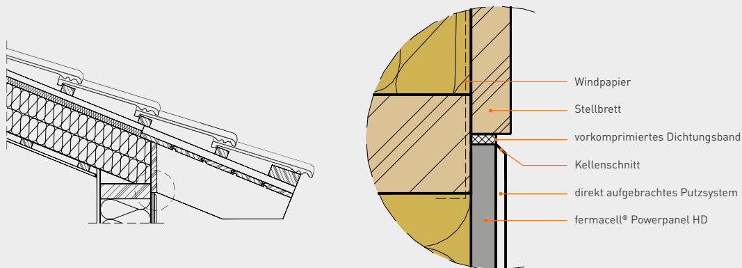
Dachanschluss der fermacell® Powerpanel HD
