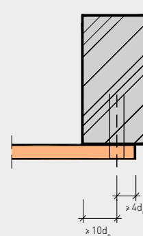
Bild 9: Abstände bei einer Randrippe/Klammern
