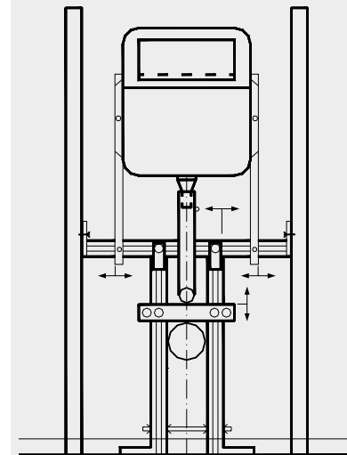
Tragständer für wandhängende WCs mit Einbauspülkästen
