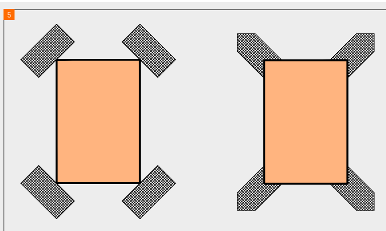
Diagonalarmierungen an Fenster- oder Türöffnungen mittels Verschnittstreifen (30 × 60 cm fermacell™ Armierungsgewebe HD) bzw. „Gewebepeilen“
