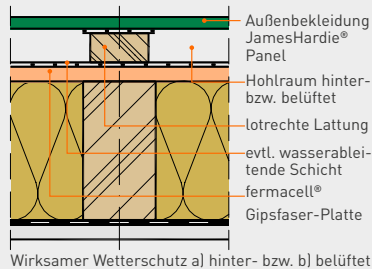
Wirksamer Wetterschutz a) hinter- bzw. b) belüftet
