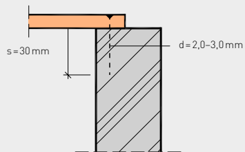
Bild 1: Nägel
