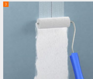
Aufrollen des fermacell™ Armierungsklebers HD
