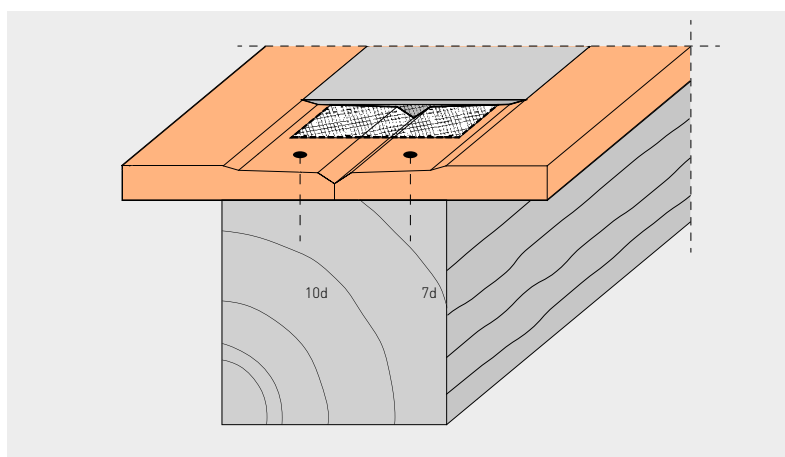
Randabstände TB-Kante für Nägel
