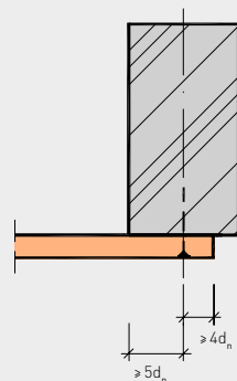
Bild 8: Abstände bei einer Randrippe/Nägel
