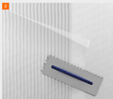
Überlappung des Armierungsgewebes mit ca. 100 mm
