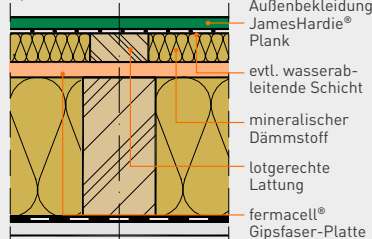
Wirksamer Wetterschutz nicht belüftet
