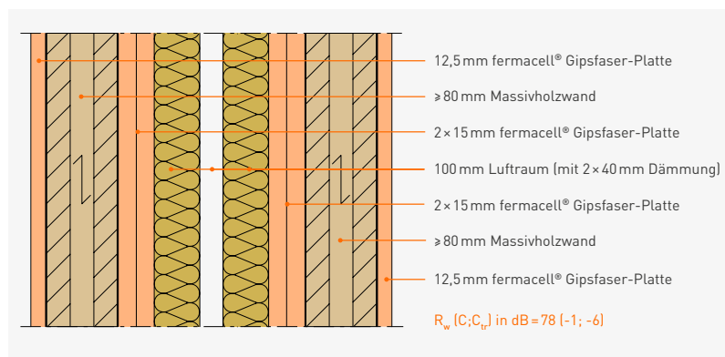
Gebäudeabschlusswand – tieffrequenter Einsatz (Beispiel)
