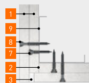
Detail 1 (mit Unterkonstruktion)
