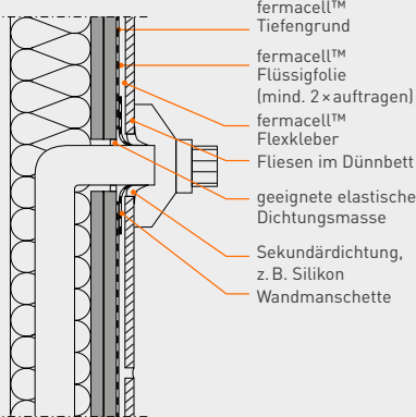
Installationsdurchführung durch Montagewand
