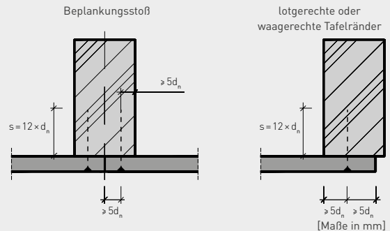
Bild 5: Erforderliche Randabstände für Nägel
