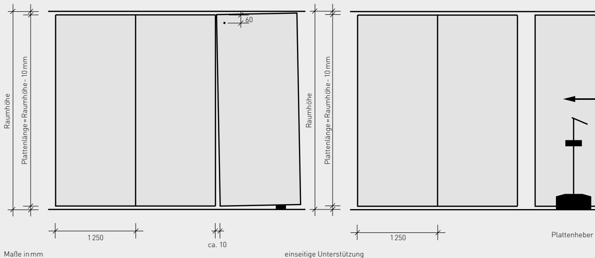
Bauseitige Montage von fermacell® Gipsfaser-Platten bei Wänden
