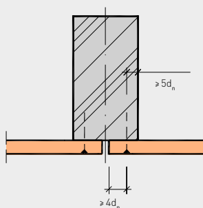
Bild 6: Abstände bei einer Mittelrippe/Nägel
