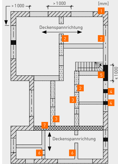
Einteilung von Wänden hinsichtlich Tragfähigkeit und Raumabschluss
