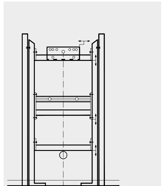
Tragständer für Waschbecken, Urinale oder Ausgüsse
