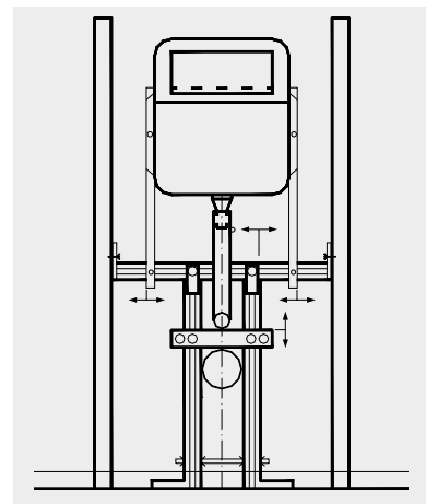
Bsp. Konsollasten: Tragständer für wandhängende WCs mit Anbauspülkasten
