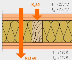
Beispiel Gebäudeklasse 4: Ausführung einer Holzständerwand (REI 60/K 2 60) gemäß den Anforderungen der Muster-Richtlinie (M-HFHolzR)/hochfeuerhemmendes Bauteil
