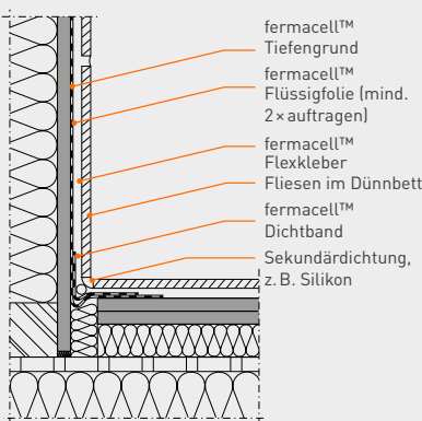
Boden-Wand-Anschluss
