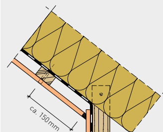
Decke an Wand
