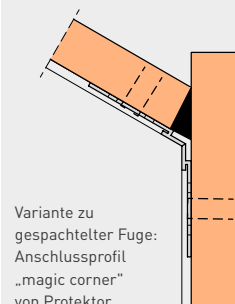
Dachschräge an Drenpel/ Abseitenwand
