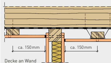
Decke an Wand
