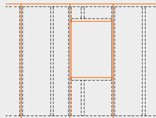
Fensteröffnung bei vertikalem Beplankungsstoß ohne Fugenversatz
