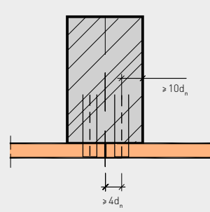
Bild 7: Abstände bei einer Mittelrippe/Klammern
