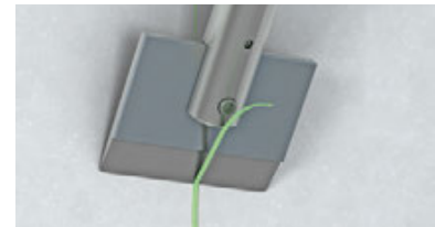
Entfernen des überschüssigen Klebers mit fermacell™ Klebstoffabstoßer
