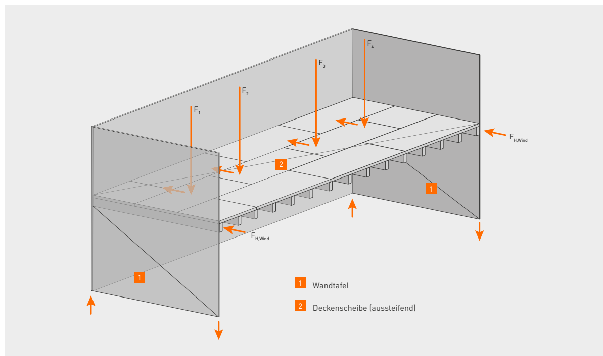
Lasteintrag (Wind) aus Deckenscheibe in seitliche Wandtafeln
