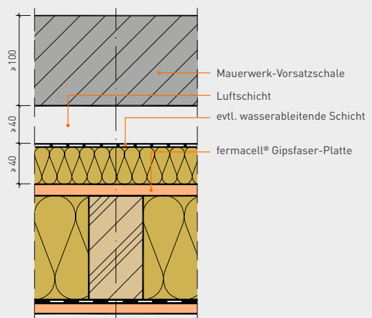
Dauerhaft wirksamer Wetterschutz Mauerwerk-Vorsatzschale
