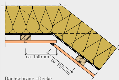
Dachschräge - Decke
