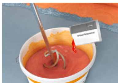
Abb. 7: 2. Auftrag: Farbkonzentrat zur Restmenge der Flüssigfolie geben und homogen einrühren. Eingefärbte Flüssigfolie satt auftragen. Weitere Informationen sind im Produktdatenblatt zu finden. Es ist empfehlenswert, den zweiten Anstrich quer zum Ersten aufzutragen, um evtl. Fehlstellen in der Abdichtungsschicht zu vermeiden.
