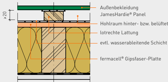
Dauerhaft wirksamer Wetterschutz a) hinter- bzw. b) belüftet
