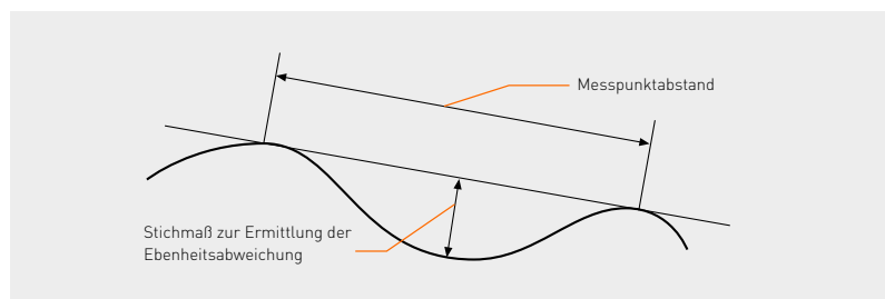
Zuordnung der Stichmaße zum Messpunktstand
