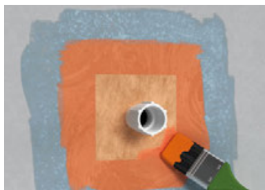
Abb. 4: Zur Abdichtung von Rohrdurchführungen die fermacell™ Wanddichtmanschette in die noch feuchte fermacell™ Flüssigfolie einbetten und direkt erneut überstreichen – Trocknungszeit mind. 1 Stunde
