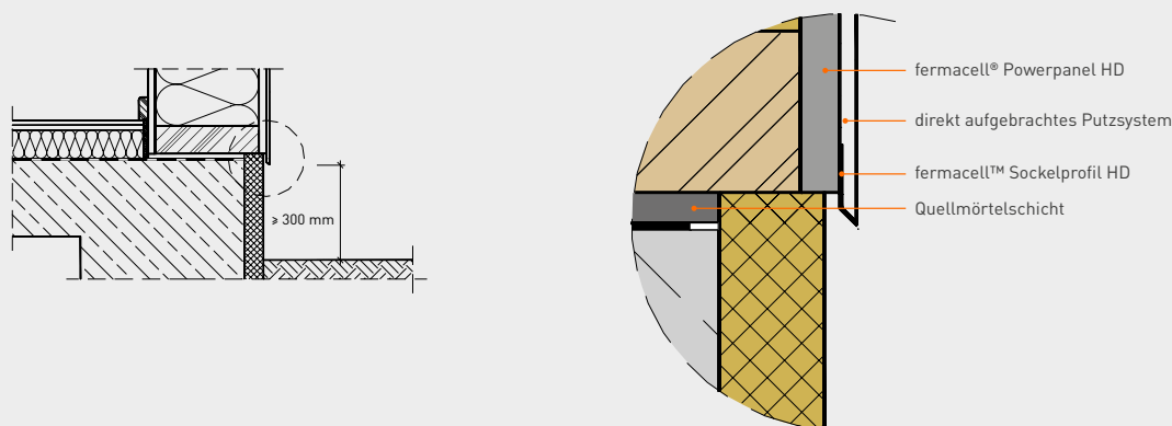
Anschluss der fermacell® Powerpanel HD im Sockelbereich
