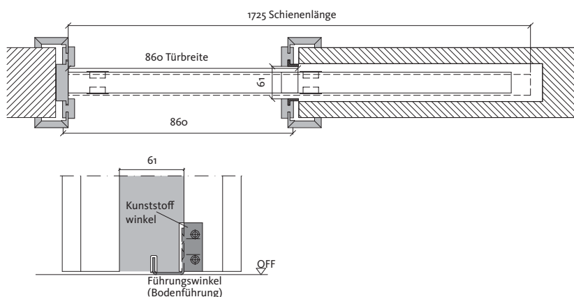
In der Wand, im Sturz Konstruktion B
