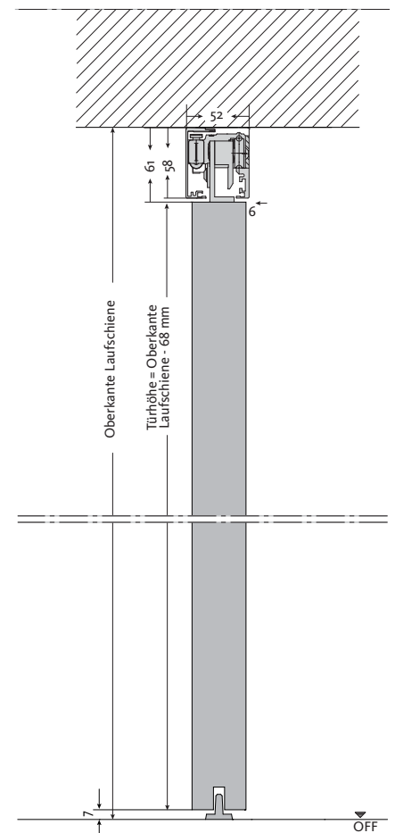
ohne Zarge Deckenmontage
