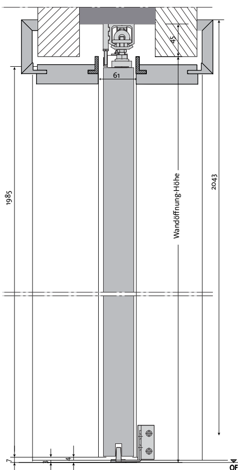
In der Wand, im Sturz Konstruktion B
