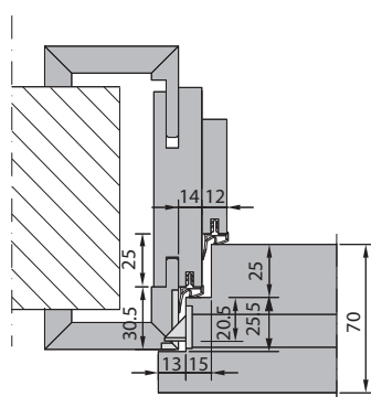
Tür 70 mm Doppelfalz
