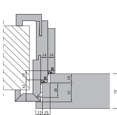
Tür 70 mm Doppelfalz, WE 68 RC3
