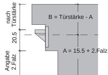
Tür mit Doppelfalz (Angabe 2. Falz)
