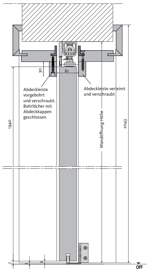
In der Wand, unterm Sturz Konstruktion A
