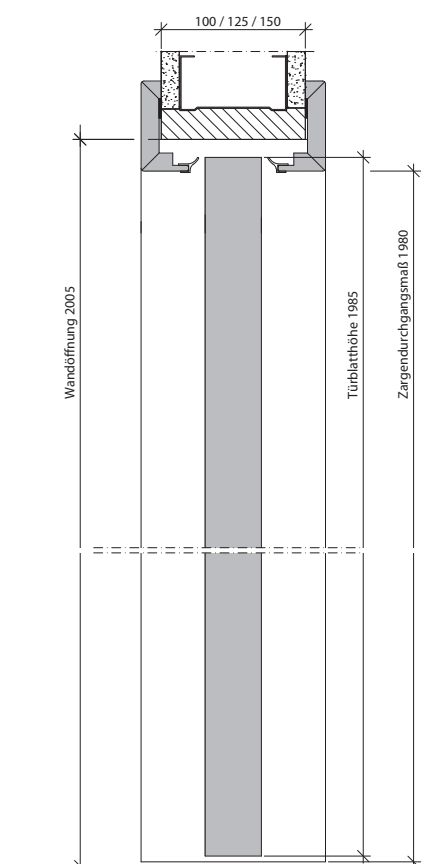
Abbildung: SE II Systemkasten Holz Tür- und Durchgangsmaß bei Glas identisch.
