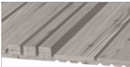
Gestaltungsvorschlag 1: 3x 40x68 mm, 3x 21x146 mm
